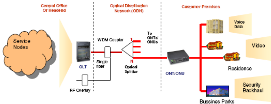
Gambar 1. Arsitektur Layanan Umum Passive Optical Network (PON)
