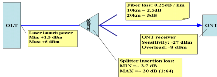
Gambar 2. Persyaratan sinyal pada GPON
